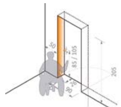
Türmaße
